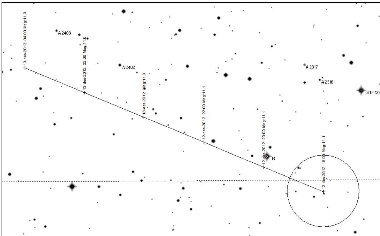
Asteroiden 4179 Toutatis 12.des. 2012 kl. 18:00 - 13. des. kl. 04.00. Sirkelen er omtrentlig feltstørrelse med 40mm Pentax XW okular på TAF C14 teleskop.
