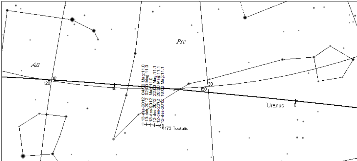
Asteroiden 4179 Toutatis 12.des. 2012 kl. 18:00 - 13. des. kl. 04.00. Oversiktskart.
