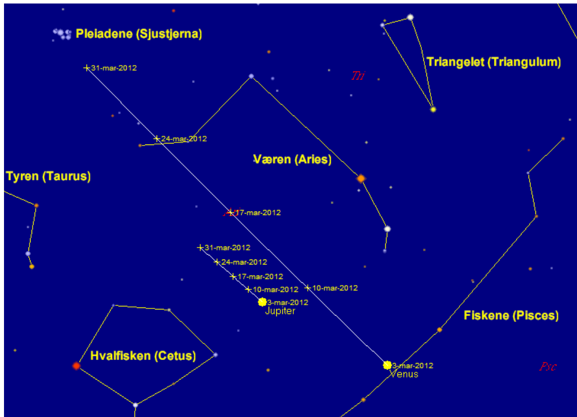
Venus passerer Jupiter i mars 2012. Posisjoner inntegnet for hver 7. dag de neste fire ukene.
